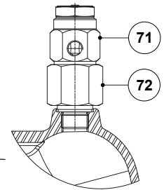
Optionaler Vakuumbrecher (VB21M)
