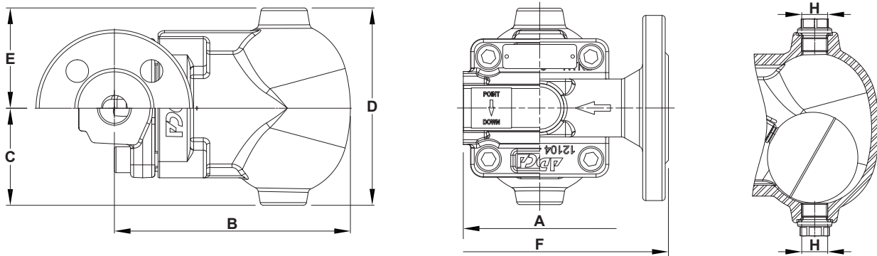
Inline-Konstruktion
