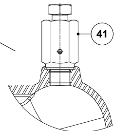
Optionales Manuelles Entlüftungsventil (HVV)
