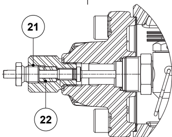
Optional Bypass-Ventil gegen Dampfabschluss (SLR)
